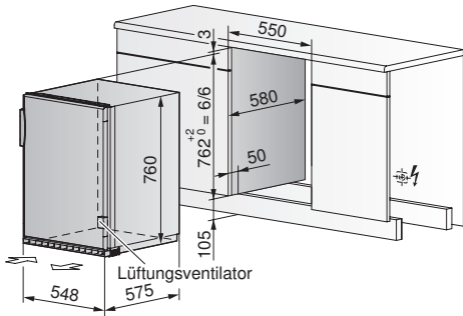
Réfrigérateur à encastrer norme SMS / 55 cm 6 / 6 Komfort
